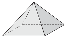
PYRAMID
